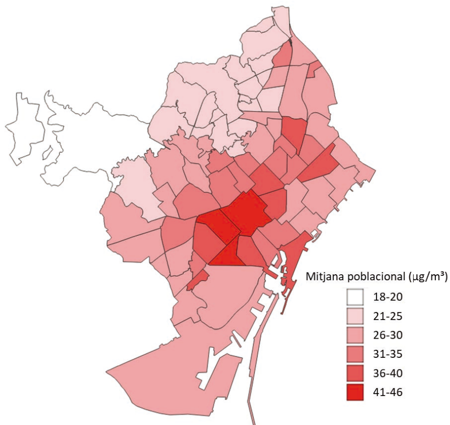
Figura 21. Mitjana poblacional d'NO 2 als barris de la ciutat, l'any 2022.
