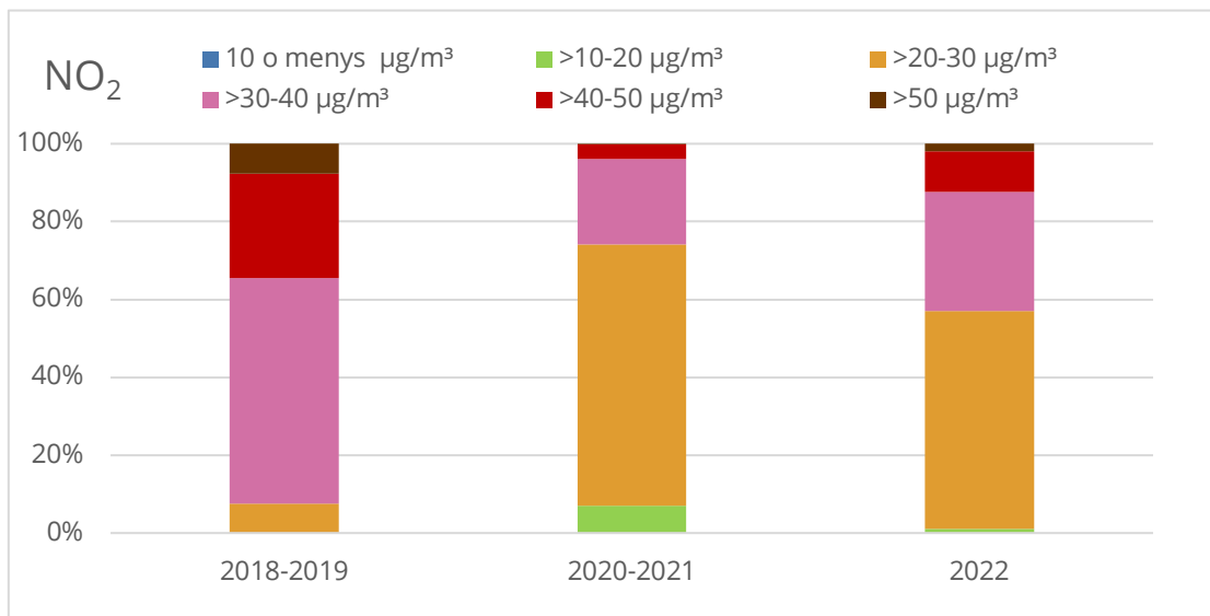
Figura 20. Percentatge de població exposada a diferents intervals d'NO 2 (µg/m 3 ) durant els períodes 2018-2019, 2020-2021 i l'any 2022.
