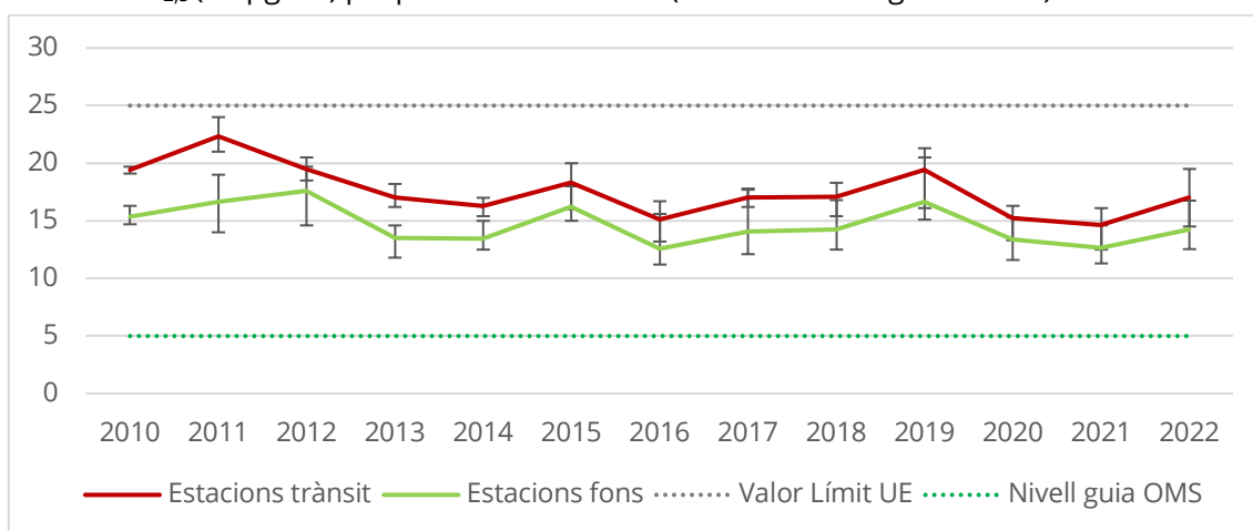
Figura 13. Evolució temporal de la mitjana anual agregada per estacions de trànsit i de fons de PM 2,5 (en µg/m 3 ) pel període 2010-2022. (Dades mètode gravimètric)
